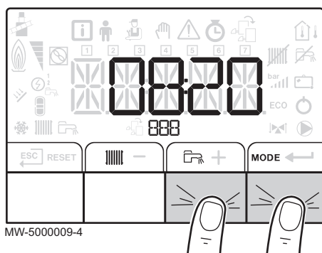
Afb.53 Handbedieningsmenu openen
