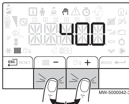
Afb.54 Richttemperatuur instellen
