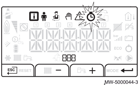
Afb.56 Circuit selecteren
