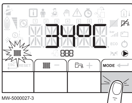
Afb.34 Uitzetmodus selecteren
